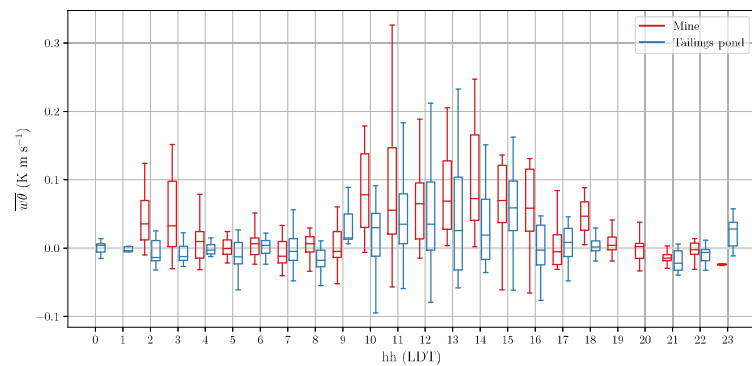
(d) Vertical kinematic sensible heat flux
